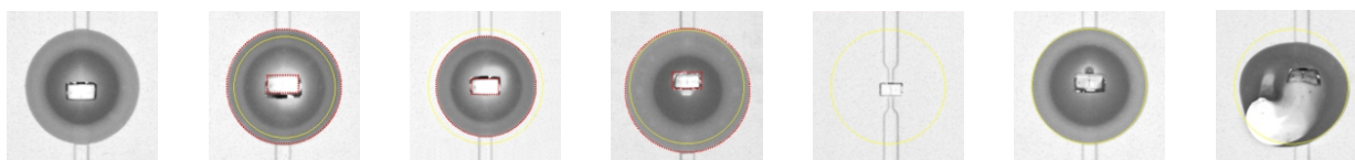
▲良品 ▲多胶 ▲少胶 ▲偏移 ▲漏胶 ▲气泡 ▲胶体不成圆
