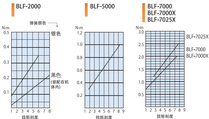
输出扭矩刻度表 (HI输入时)
